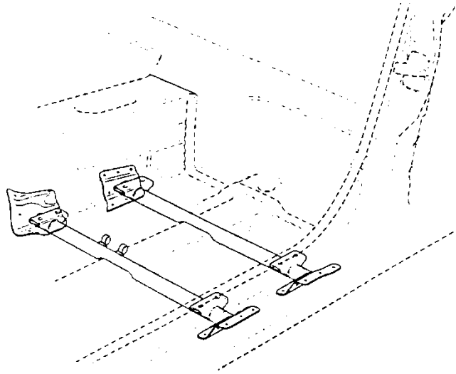
Крепление сиденья.
