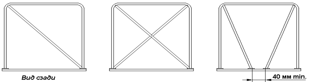
Рис. 6. Опоры каркаса, установленного внутри кабины, на автомобилях с несущей рамой.
