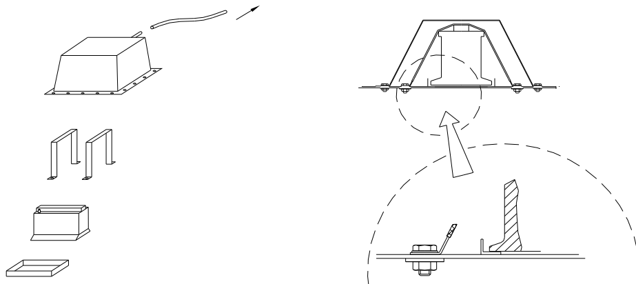
Крепление аккумулятора.
