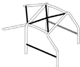
Минимально необходимая схема.
