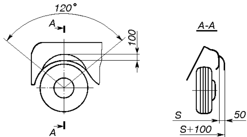
Изменение крыла легкового автомобиля.
